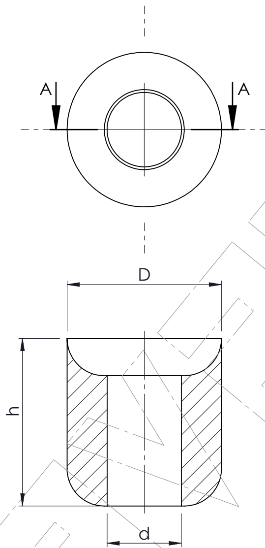
SEZIONE A-A
